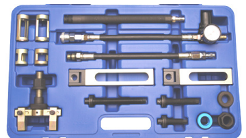
BGS8475 Klep-veerlichter zonder de cilinderkop te moeten demonteren Lève-soupapes universel sans démonter la culasse. European, American, Japan cars. Mercedes M102-103-104-111-112 M113-271-272 / BMW N42-52-62-M54- M52-M56, E38, M60, V8
